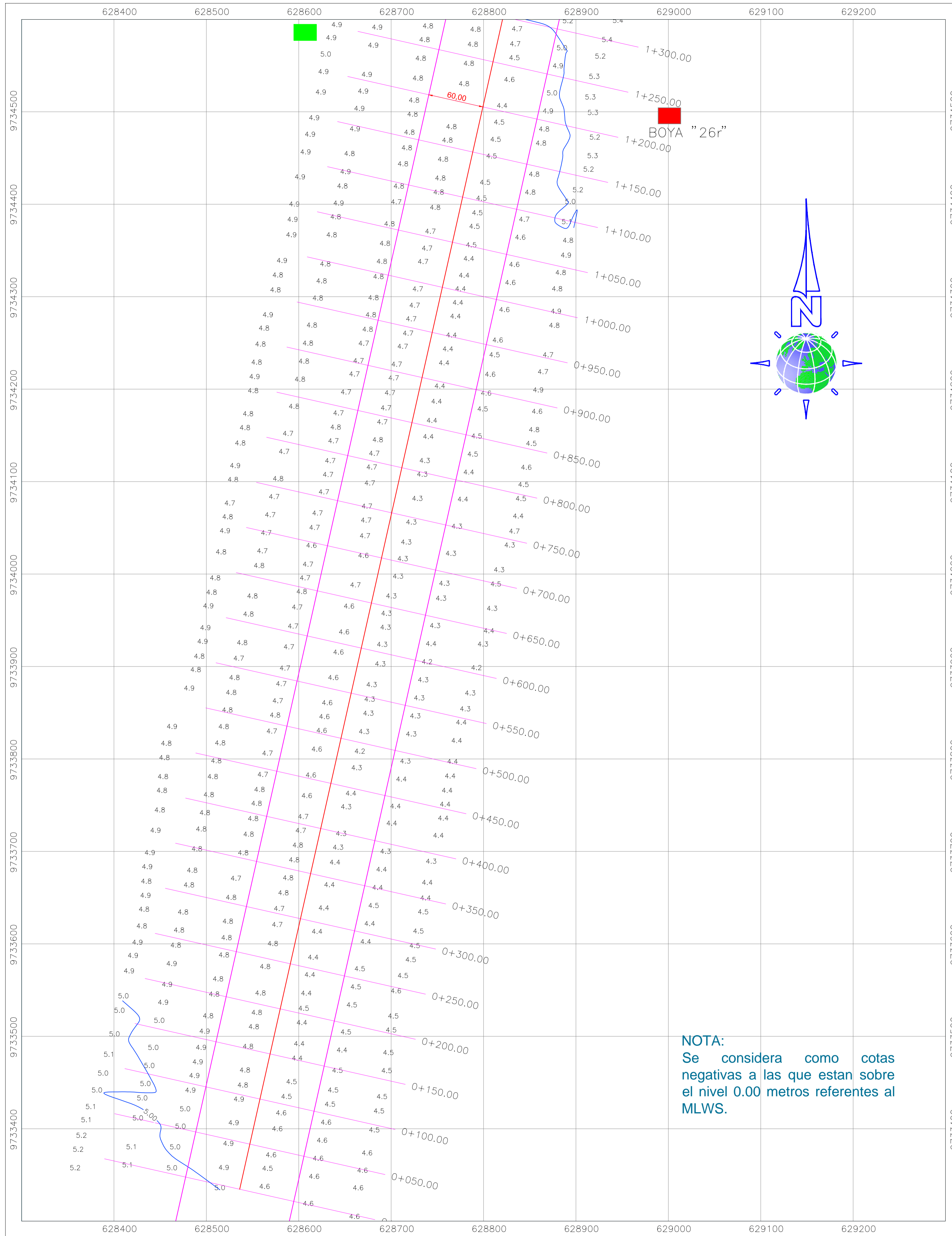
PLANTA BATIMETRICA ESCALA 1 : 2500
